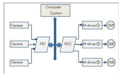
図 位置決め装置のCPUモデル
